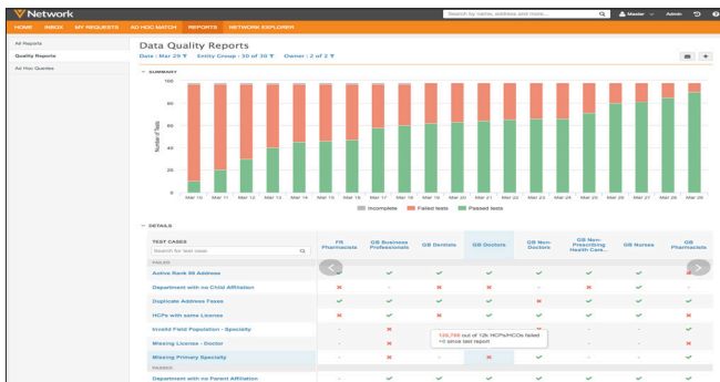
그림 2: 데이터 품질 보고서의 품질 추세
